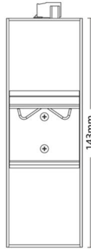
نمای پشت
