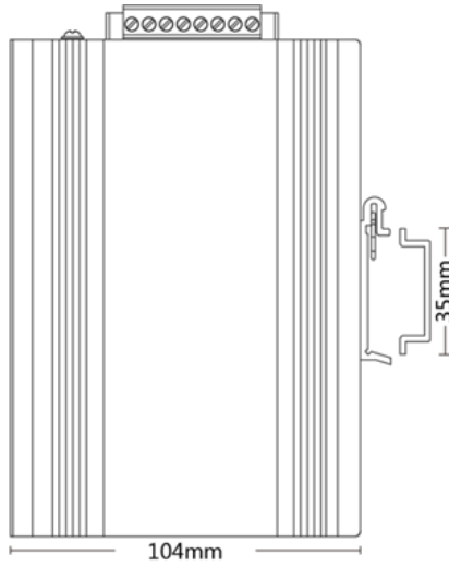
نمای جانبی
